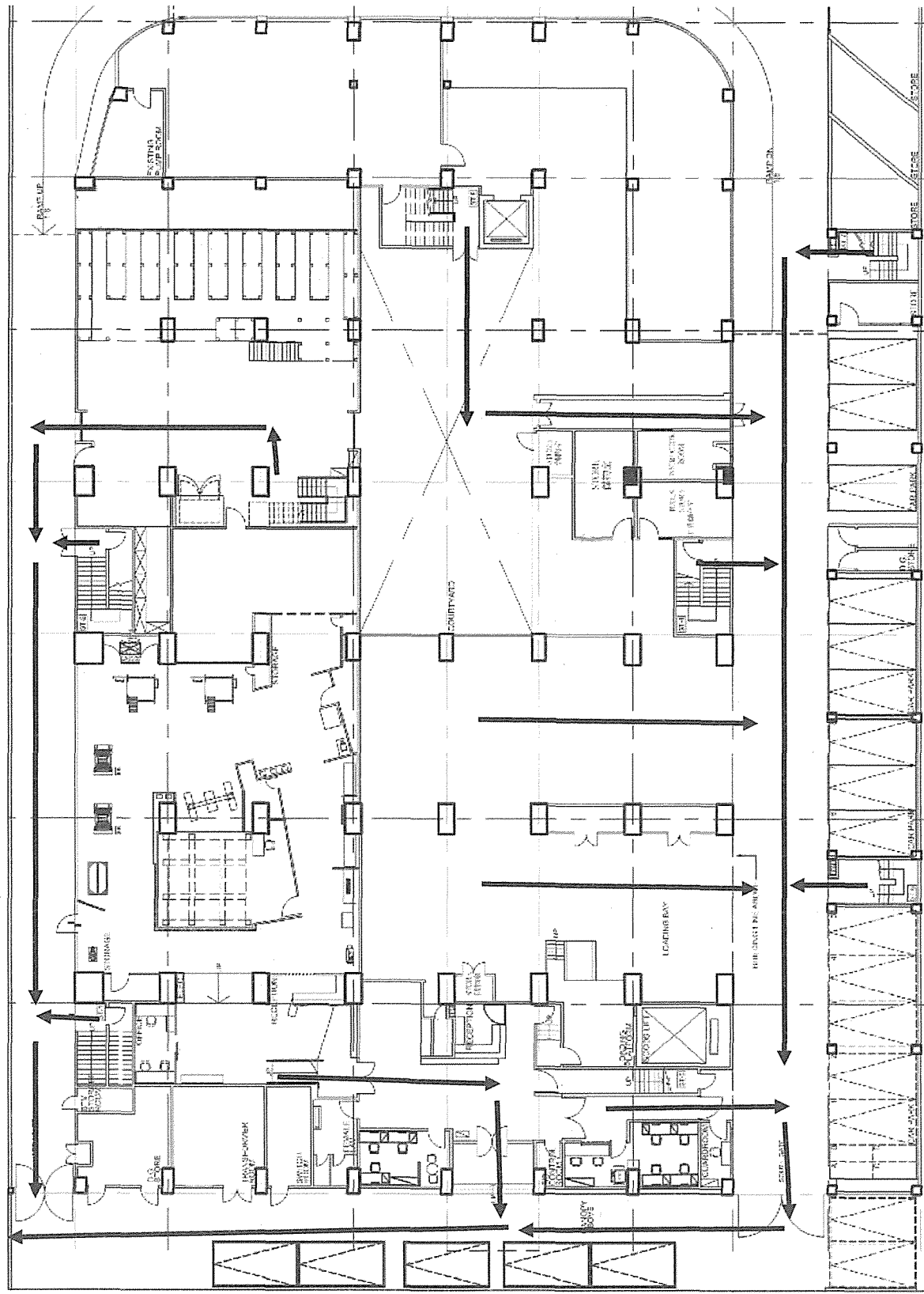
GROUND FLOOR FIRE ESCAPE ROUTE LAYOUT PLAN 地面火警逃生路線圖
